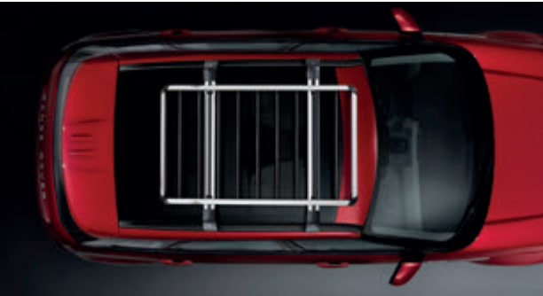
行李架 *Δ LR006848 灵活的行李架系统，为车顶运载提供方便。提供高达75千克的承载能力。最大有效载荷62.6千克。
