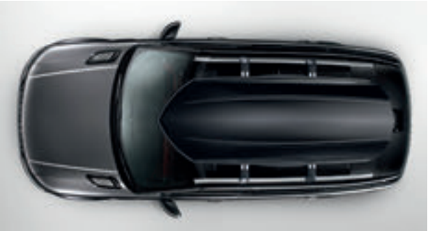
运动器材箱* VPLVR0061 大型运动器材箱* VPLVR0100 (未展示) 亮黑色活动箱外形美观时尚,符合空气动力学原理。可安装在车辆两侧,便于停靠路边时打开。内置雪橇或其他长件物品保持系统。最大容量320升,最大载荷75千克*。
