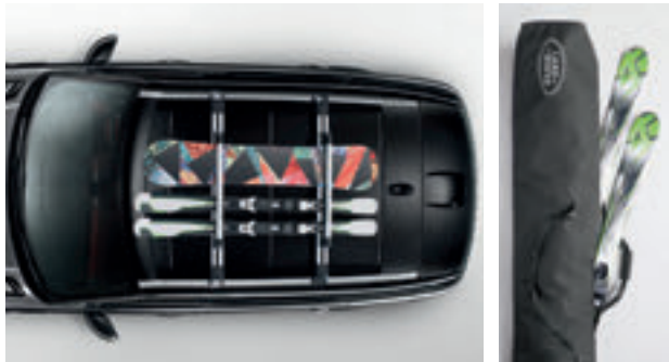
雪橇/滑雪板架* LR006849 可装载四对雪橇或两块滑雪板。提供便于装载的滑轨，可安全锁定。最大有效负荷36千克*。 雪橇袋 VPLGS0166 最多可搭载两对滑雪板和长度为180厘米的滑雪杆。由坚固耐用的600D涤纶线编制，带有可拆卸式肩带。
