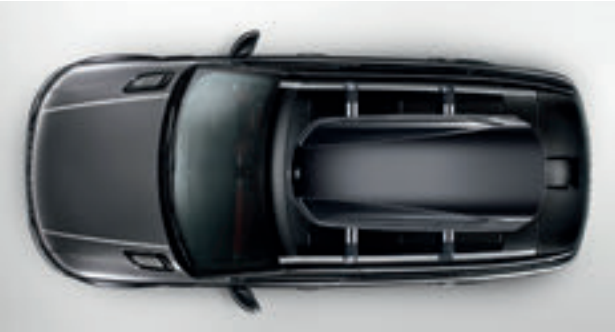
车顶行李箱* VPLVR0062 亮黑色车顶行李箱可从两侧打开,可锁定以确保安全性。包括强力夹具,可轻松快捷安装于车顶横杆上。外形尺寸:1750x820x450毫米,容量410升。最大有效载荷75千克*。
