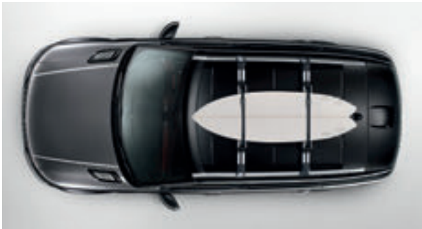
水上运动装备架* VPLGR0107 可承载一个冲浪板，帆板，皮划艇或独木舟。包括可锁定的多功能支架能携带桅杆，平桨或划桨。可倾斜，以方便装卸。具备可锁定束带和橡胶支座，保持最佳的重量分配，同时保护皮艇和车辆不被划伤刮擦。载重45千克。
