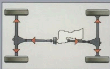
Antriebssystem 4x4 permanent
